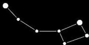
Малая медведица
