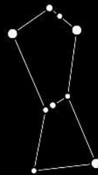
Орион
