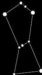
Орион
