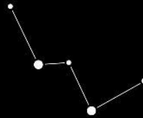
Кассиопея
