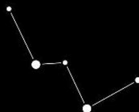
Кассиопея
