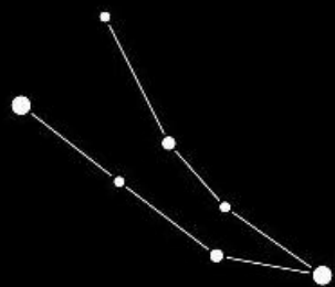
Андромеда
