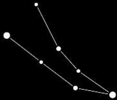
Андромеда
